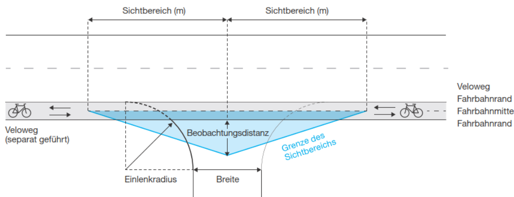
Sichtbereiche auf Velowegen (Anhang 5 VErV)
