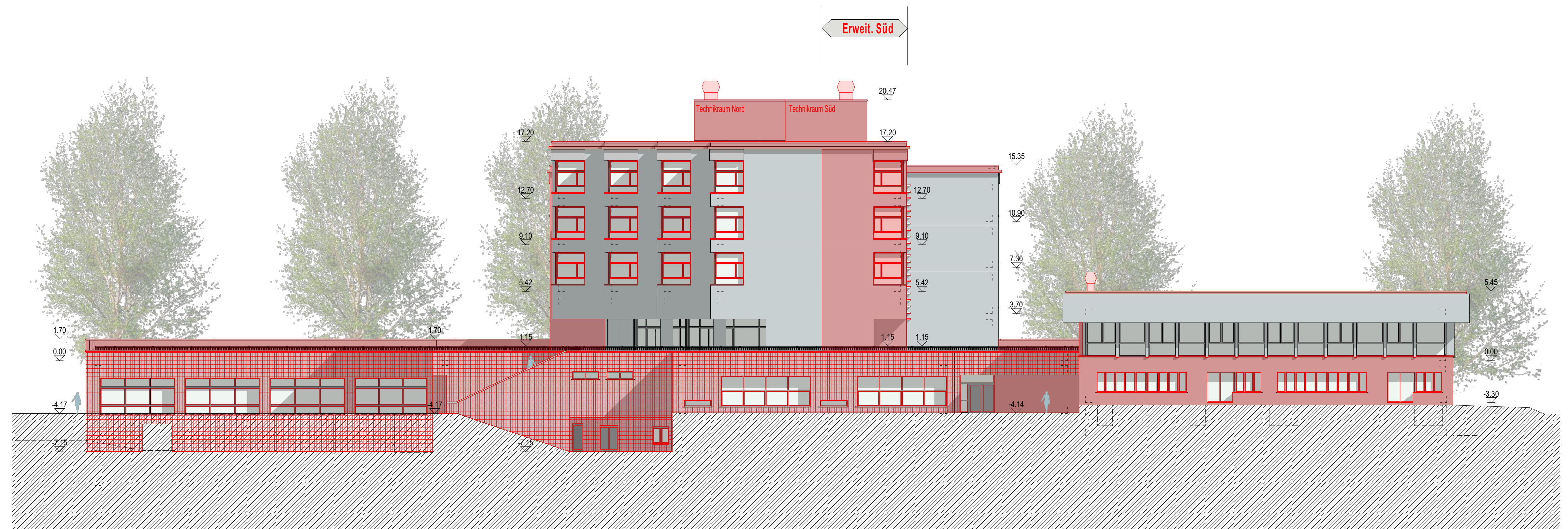
Süd Fassade Mst. 1 : 200
