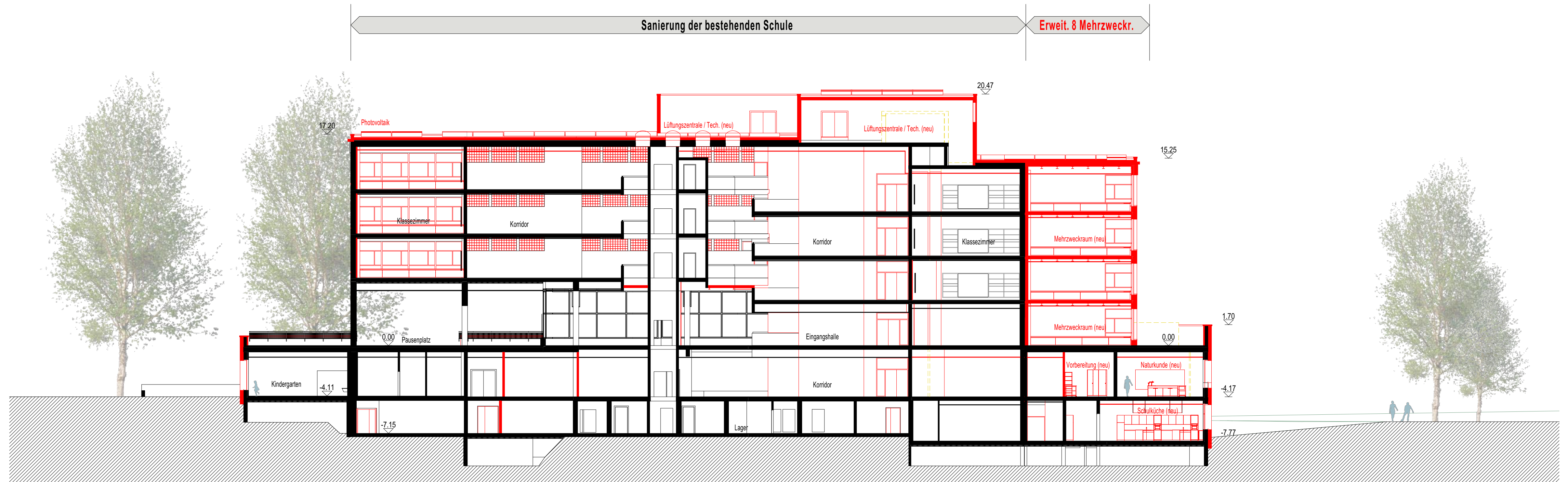
Schnitt B - B Mst. 1 : 200
