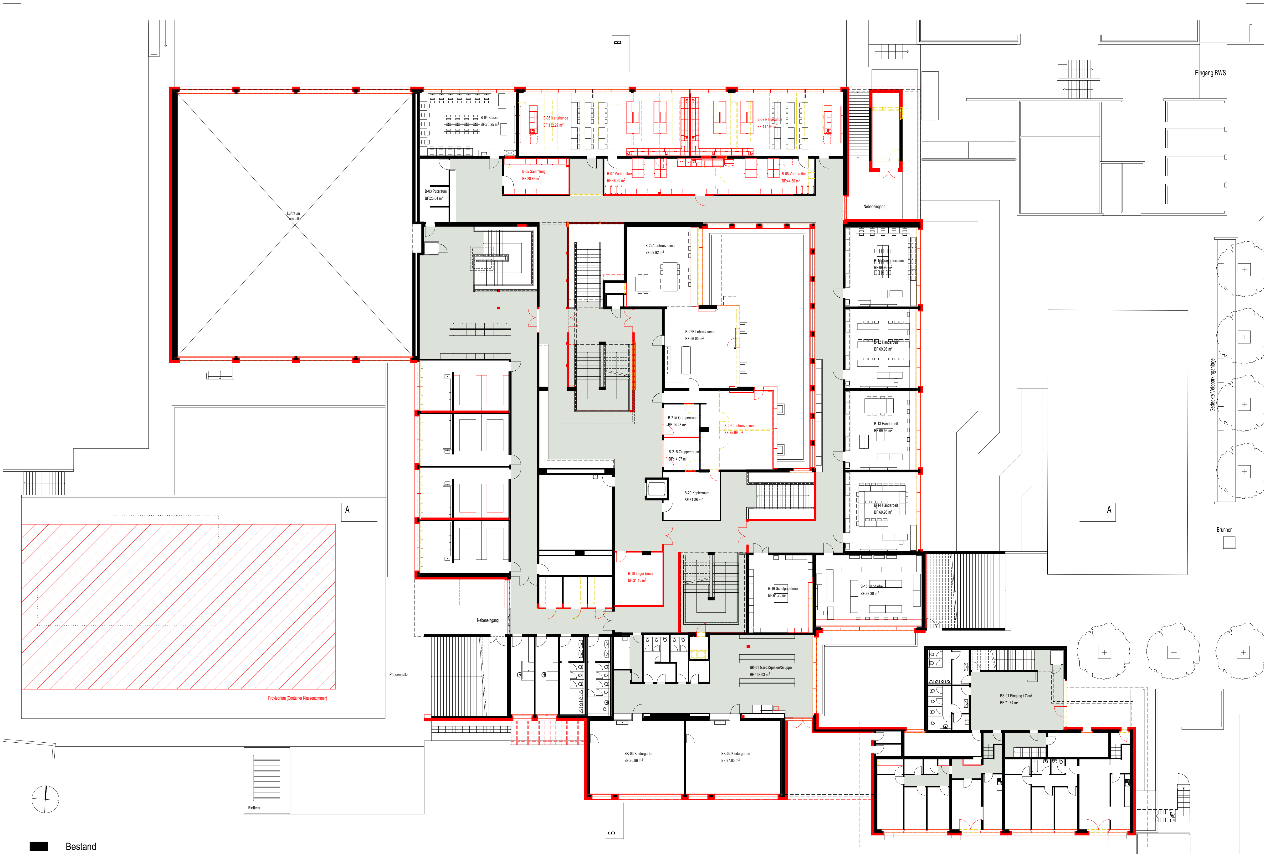
1. Untergeschoss Mst. 1 : 200
