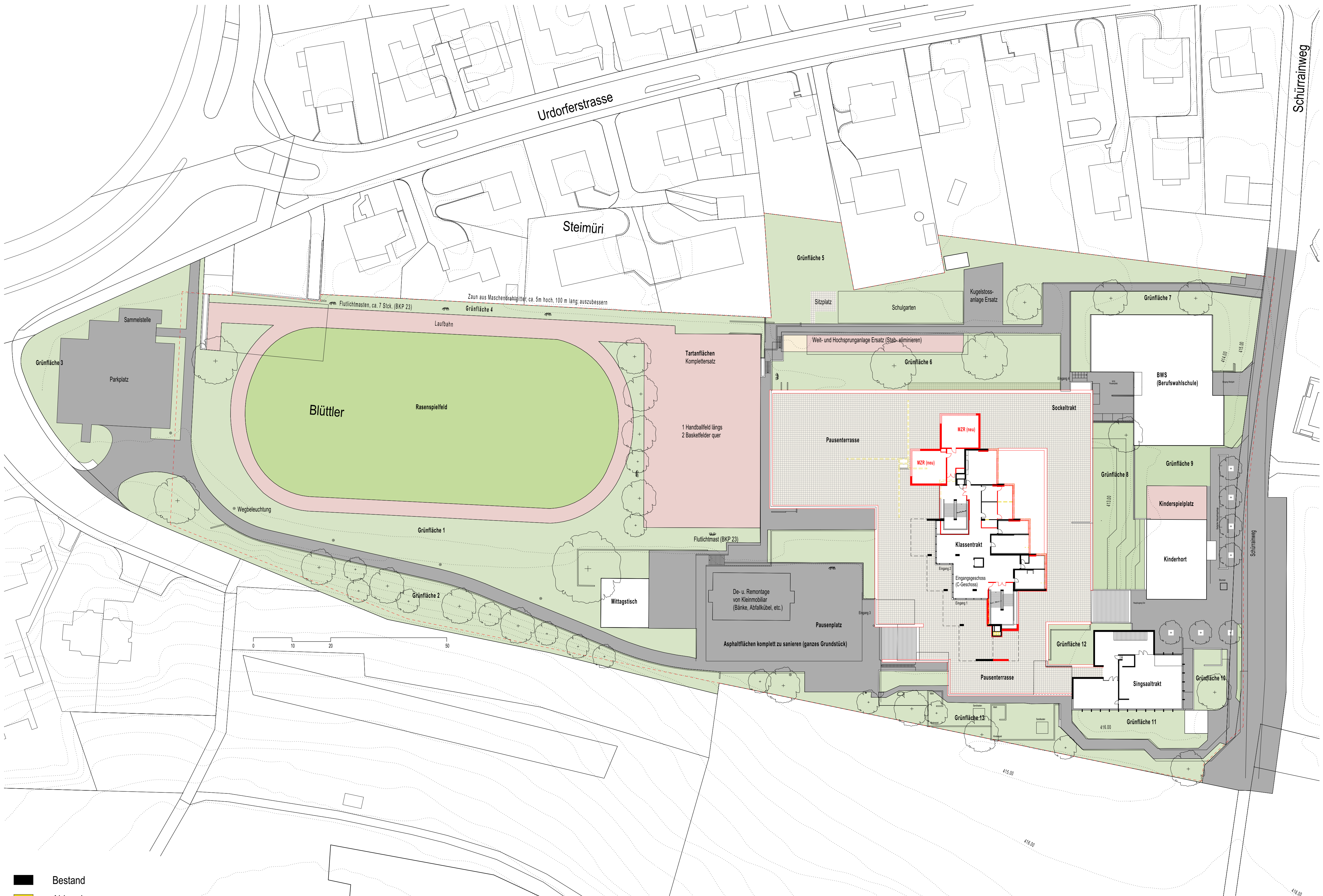
Situation Mst. 1 : 500
