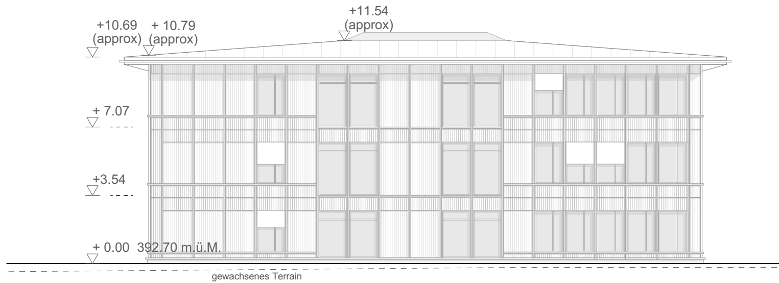
Ansicht Süd
