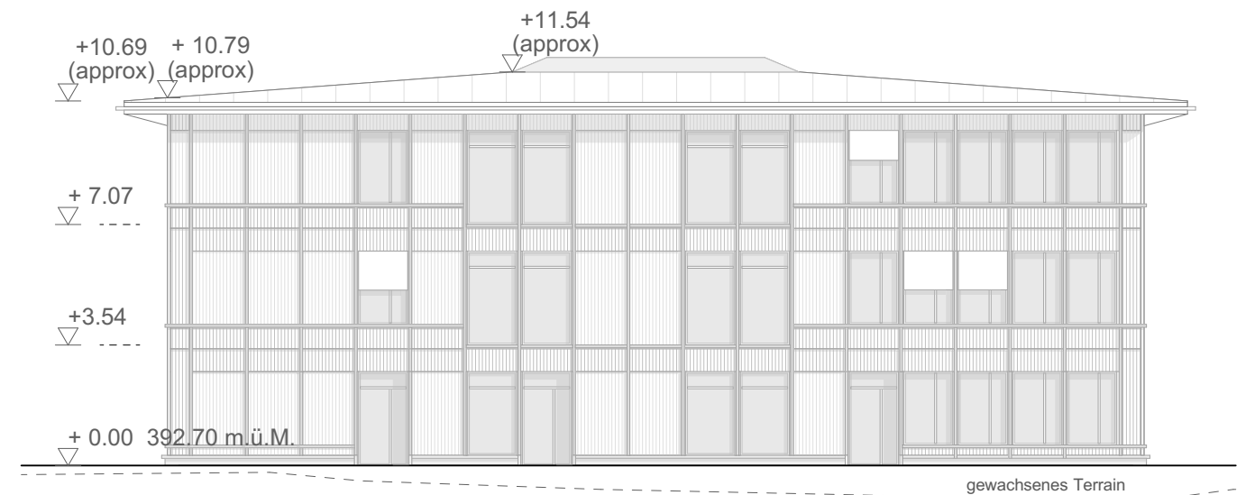
Ansicht Nord
