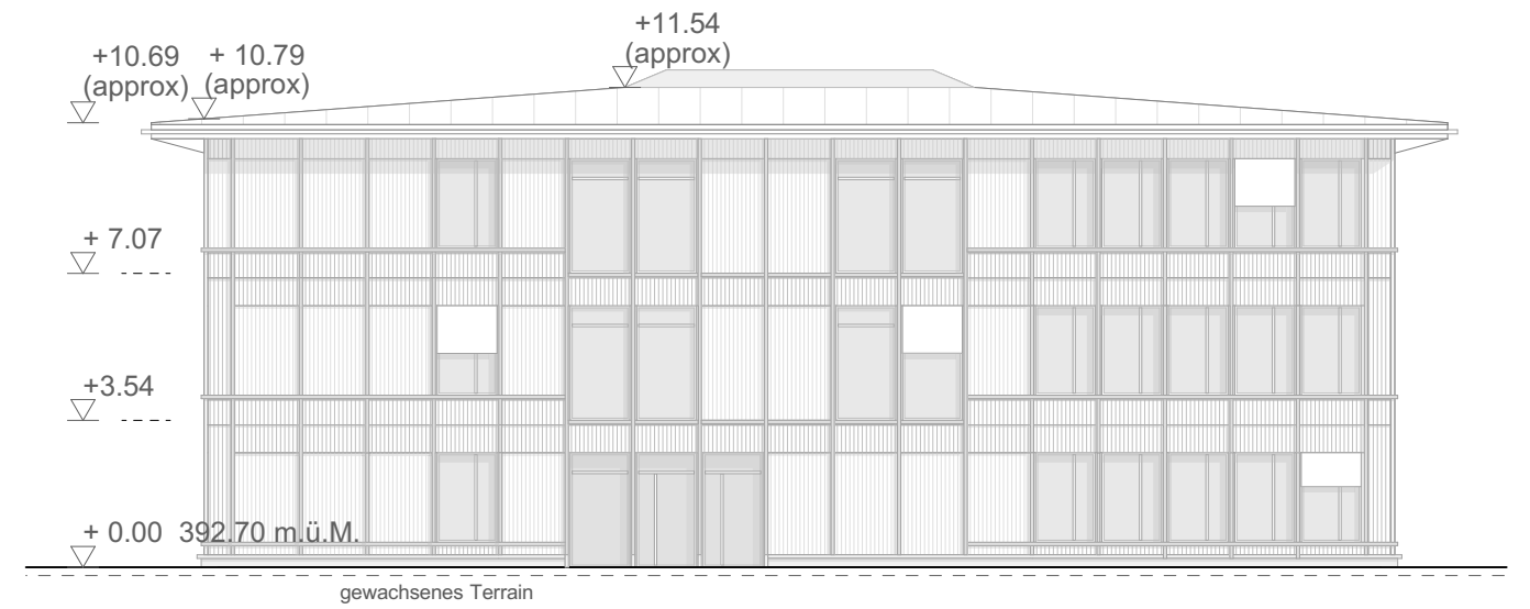
Ansicht Ost
